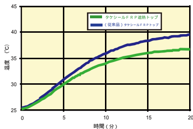
図 - 2. 遮熱試験結果
