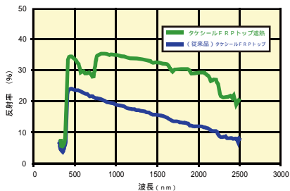
図 - 1. 分光反射率
